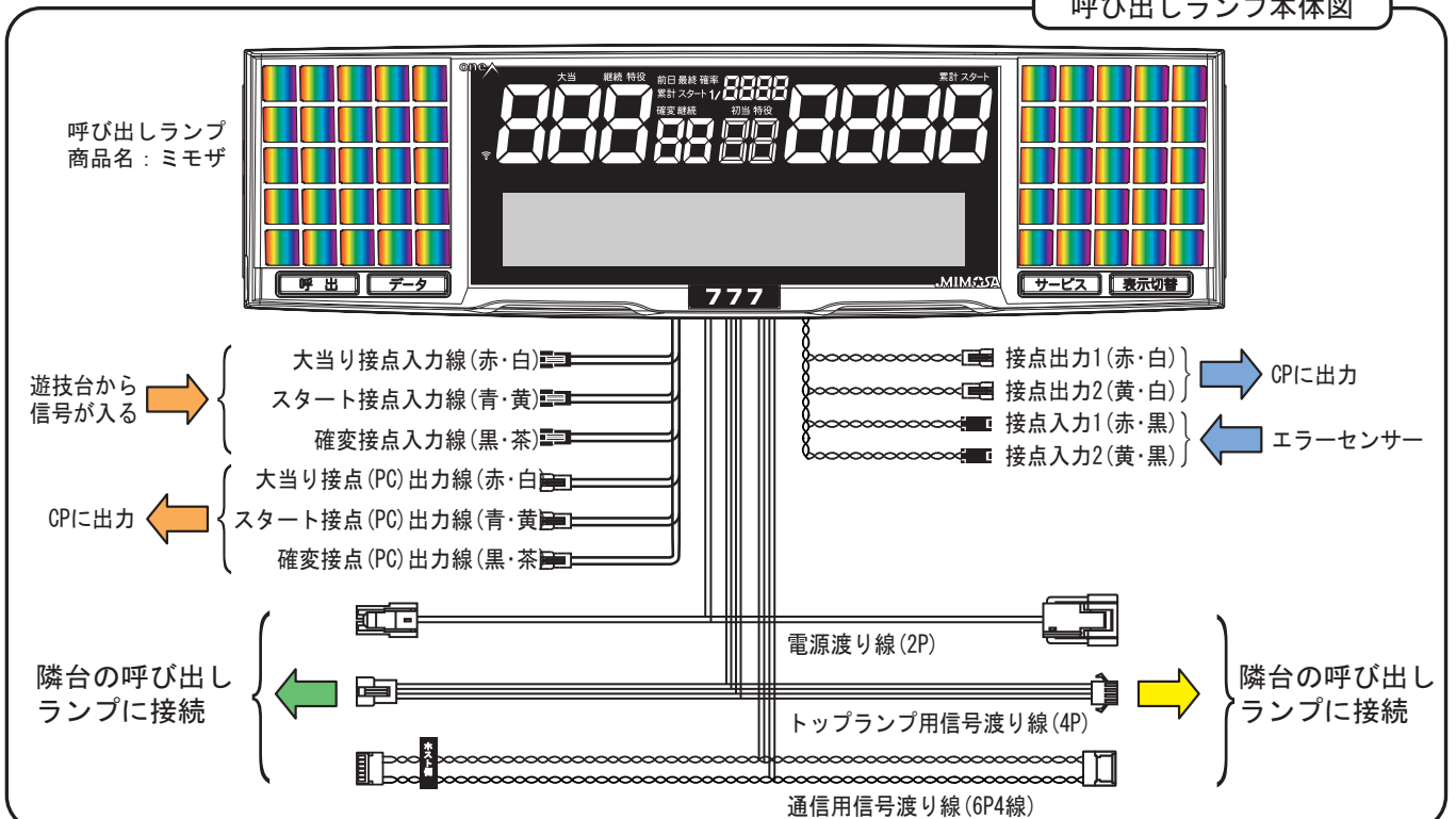
呼び出しランプ本体図
